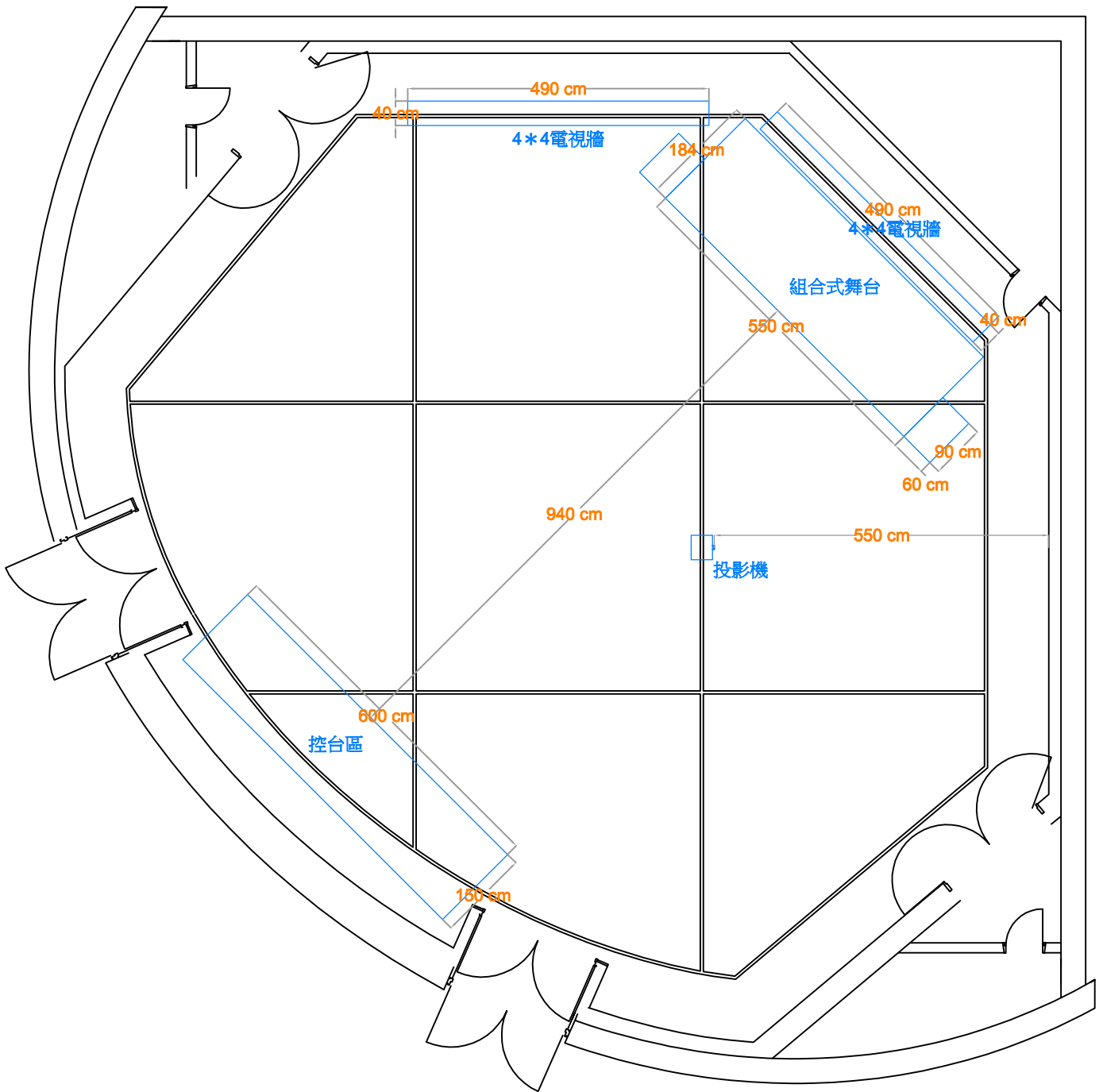
臺中國家歌劇院 角落沙龍 平面配置圖
